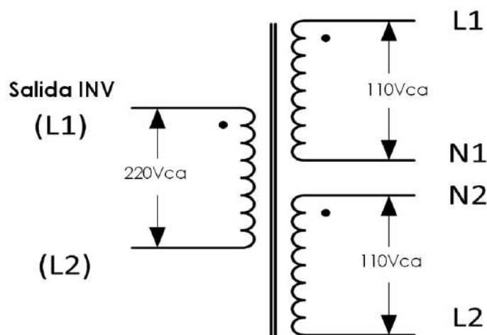
FIGURA. 2.19. ESQUEMA DEL TRANSFORMADOR DE AISLAMIENTO DE SALIDA
