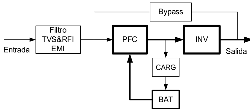
FIGURE 2.9. ESQUEMA DE MODO BATERÍA
