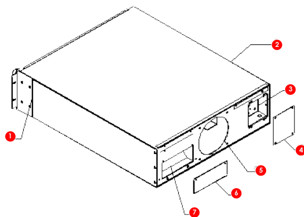
FIGURA 2.4. MÓDULO TRANSFORMADOR (6 / 10 kVA)
