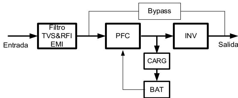
FIGURA 2.7. ESQUEMA DE MODO NORMAL (LINE)
