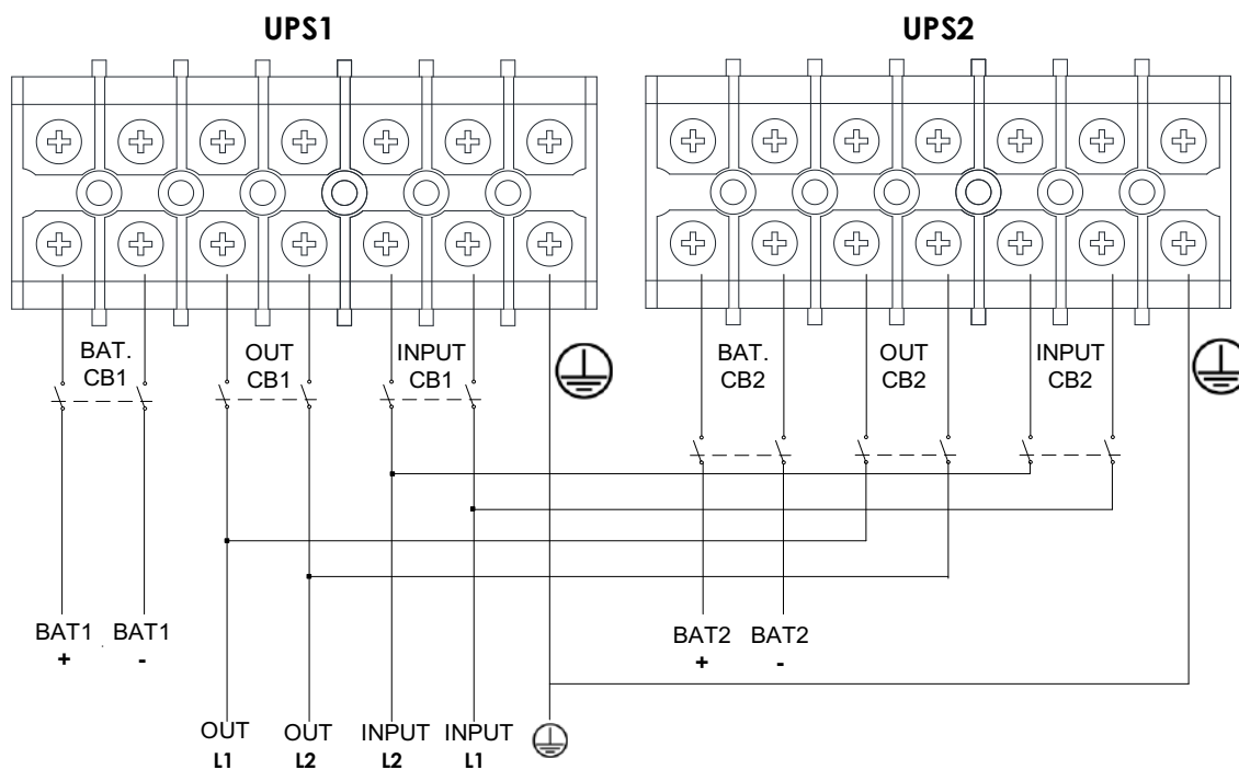
FIGURA 2.20. DIAGRAMA DE CABLEADO ELÉCTRICO DE SISTEMA PARALELO
