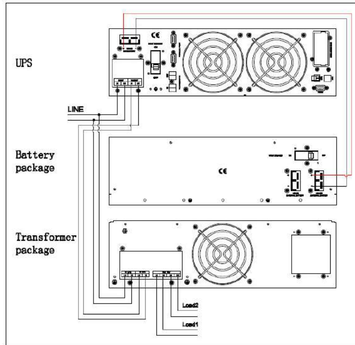
FIGURA. 2.18. CONEXIÓN DE SISTEMA UPS 6/10 kVA
