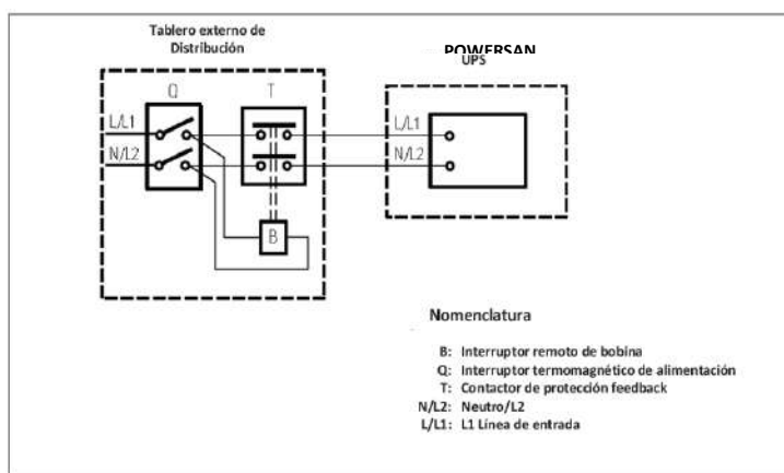
FIGURA 1.1. SISTEMA EXTERNO DE PROTECCIÓN DE RETORNO
