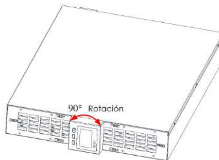
FIG.2.12. ROTACIÓN DEL PANEL LCD
