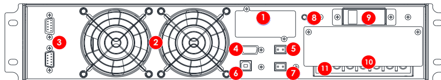
FIGURA 2.2. MÓDULO UPS 6/10 kVA (VISTA POSTERIOR)
