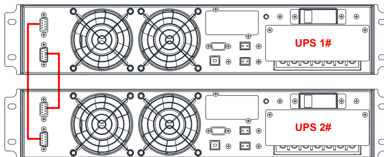
FIGURA 2.23. CONEXIÓN DE COMUNICACIÓN EN PARALELO DE 2 UNIDADES
