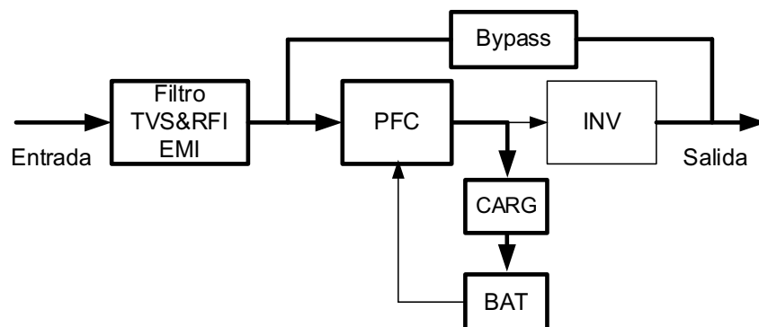
FIGURA 2.8. ESQUEMA DE MODO BYPASS ESTÁTICO
