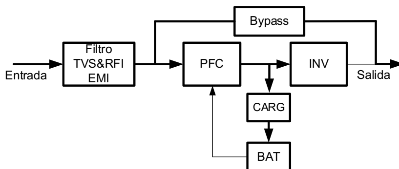
FIGURA 2.10. ESQUEMA MODO ECO
