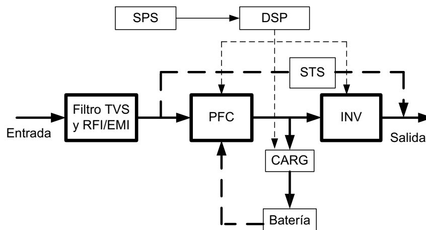
FIGURA 2.6. ESQUEMA DEL SISTEMA UPS
