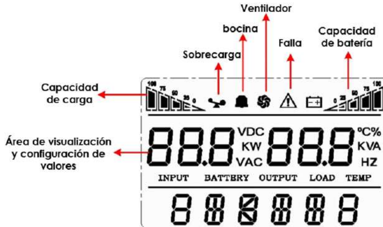
FIGURA 3.2 DESCRIPCIÓN DE PANTALLA LCD
