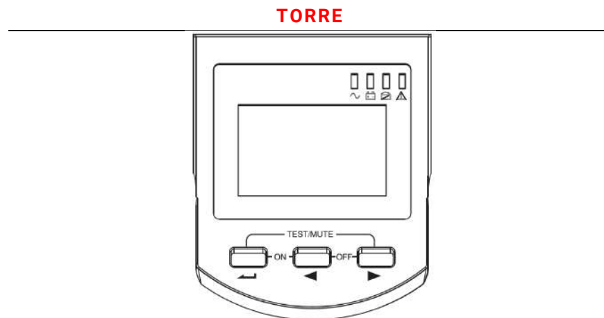
FIGURA. 3.1 PANEL DE CONTROL LCD PARA UPS 6 / 10 kVA
